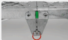
BISAGRA CON BLOQUEO CENTRAL Sistema de seguridad con pasador y anillo de bloqueo.
